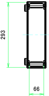
A-A (1 : 7.5)
