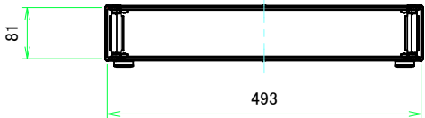
B-B (1 : 7.5)
